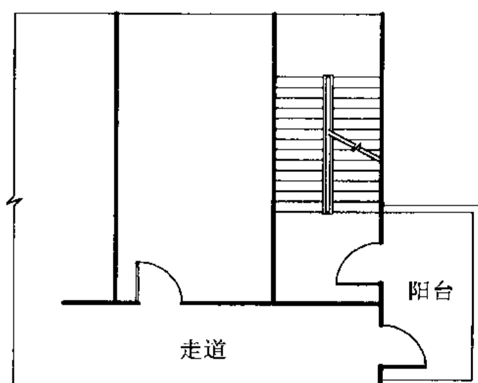
图 4.9.1-1 带阳台的防烟楼梯间
