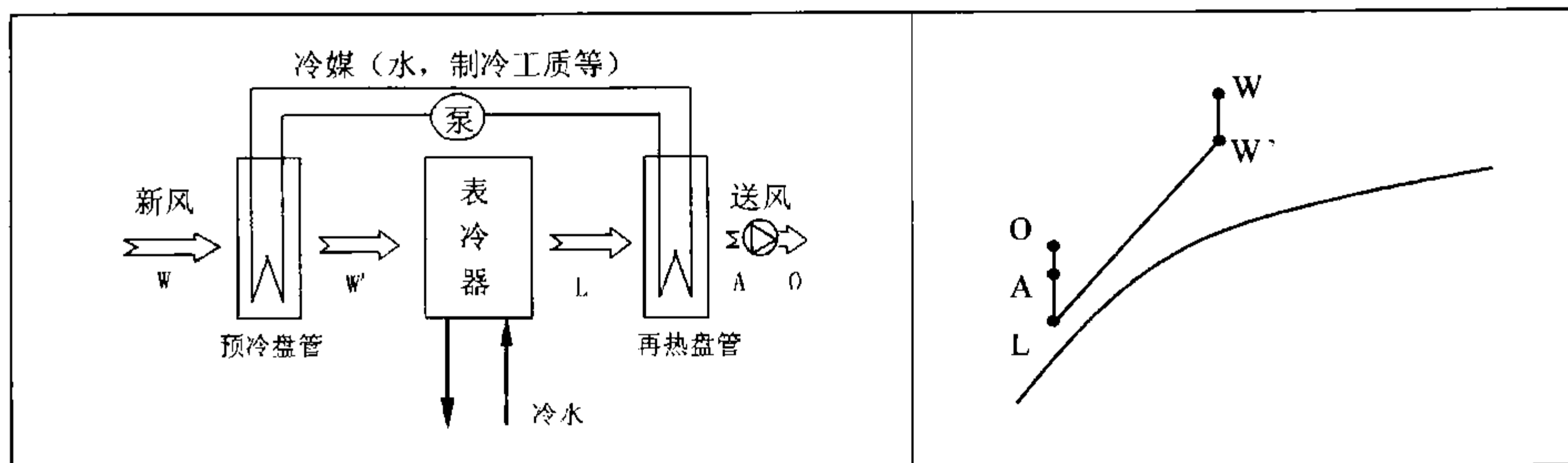
图 5.17.4-3 采用液体工质进行预冷和再热的冷却除湿系统
