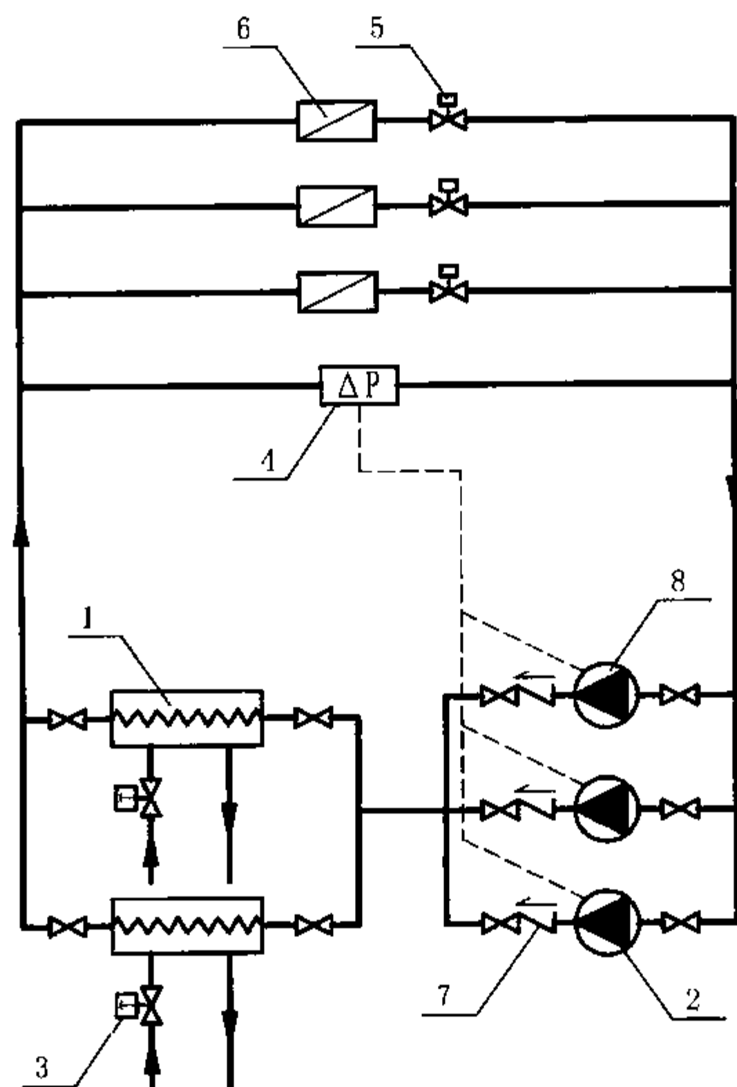
图 5.7.3-4 空调热水变流量系统示例
