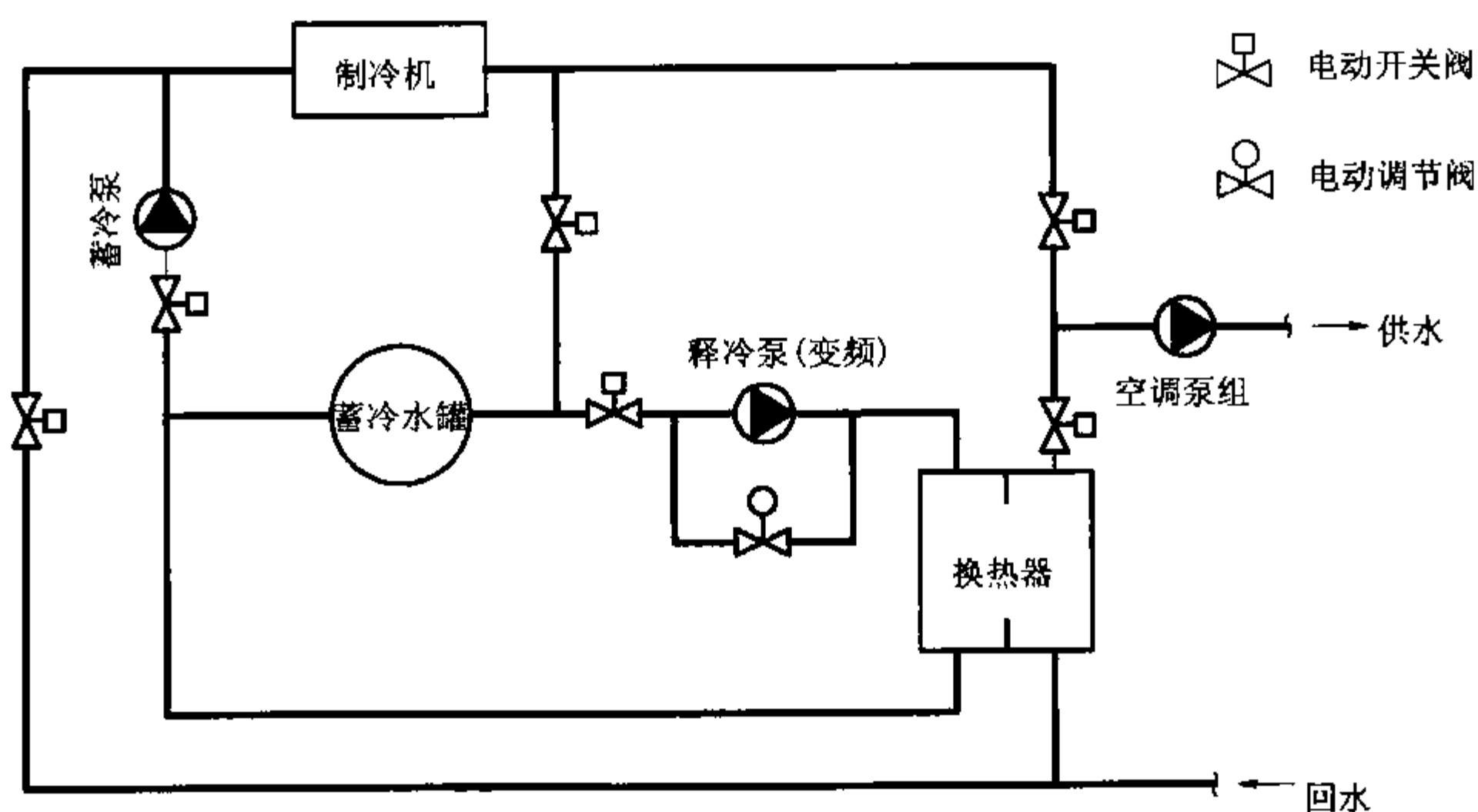
(a) 蓄冷系统内有板式换热器
