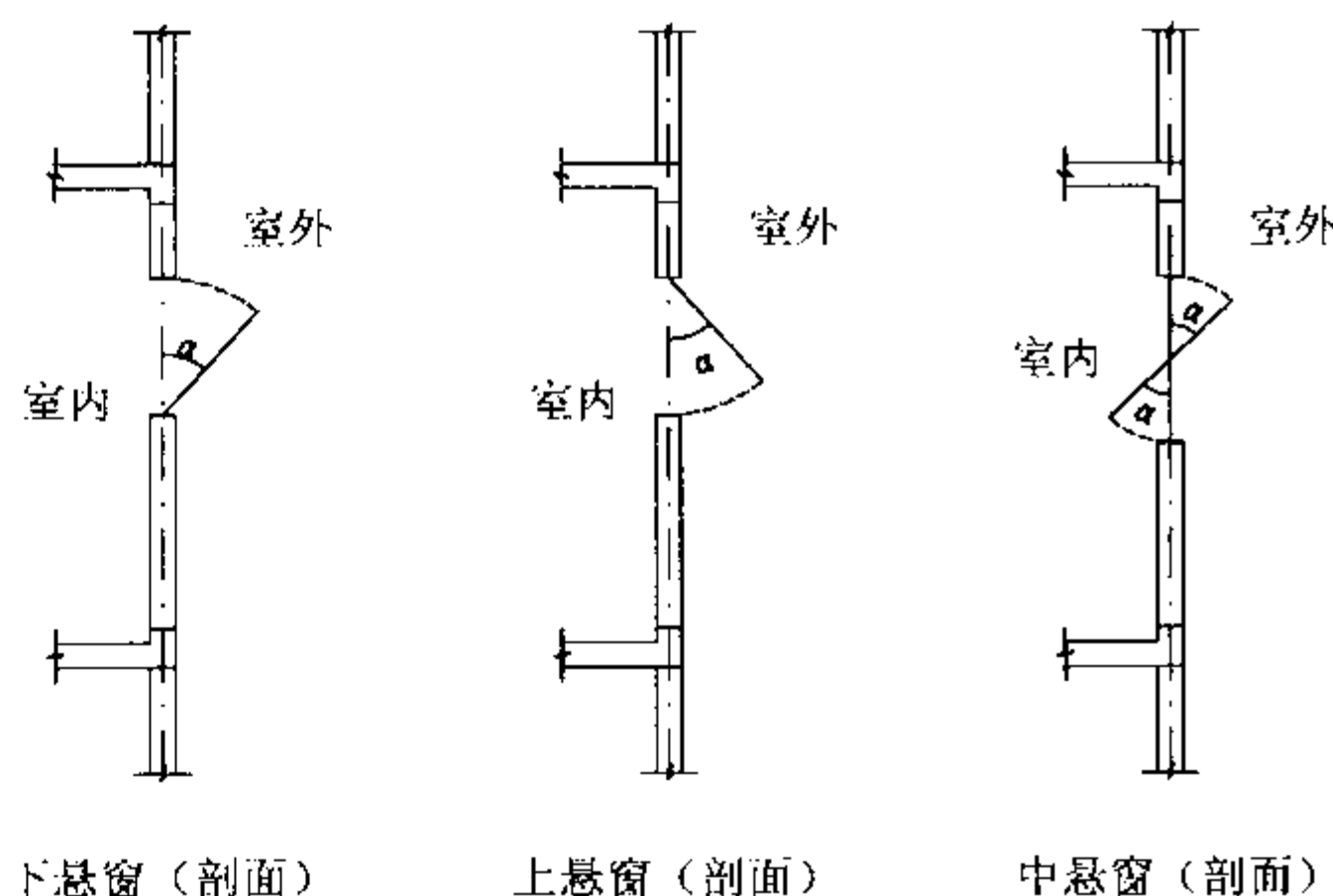
图 4.9.6 可开启外窗示意图
