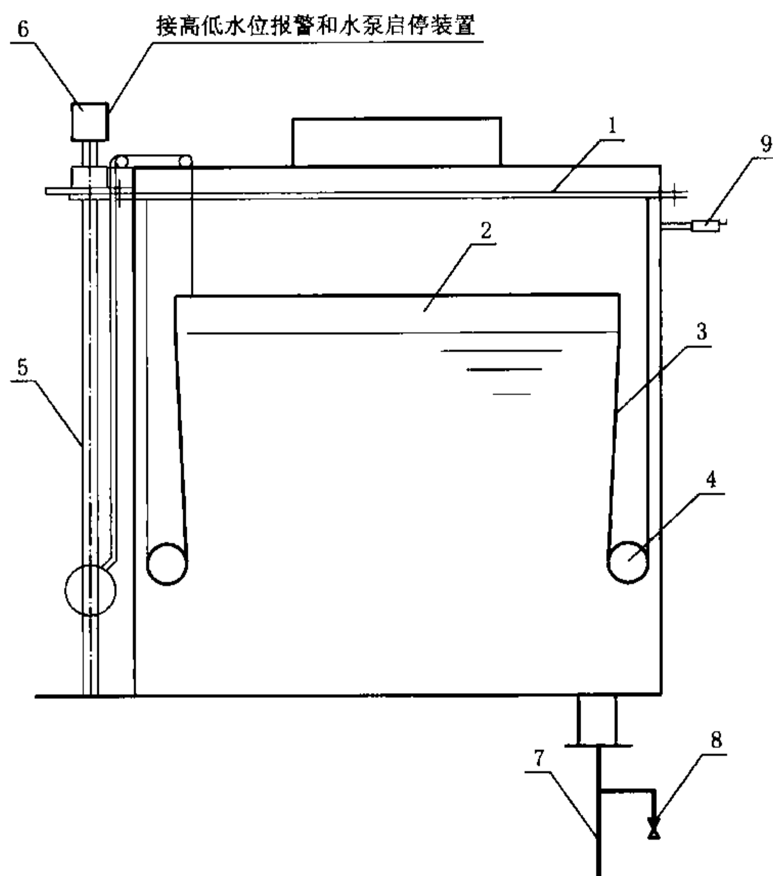
图 6.9.4 常压密闭膨胀水箱接管示意图
