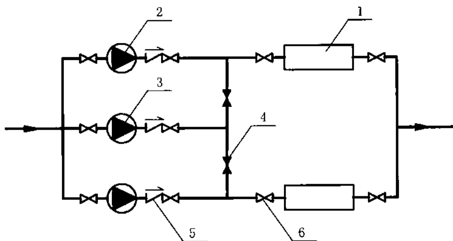
图 5.7.4-2 循环泵和冷水机组之间一对一接管连接方式（设备用泵）和阀门配置示例
