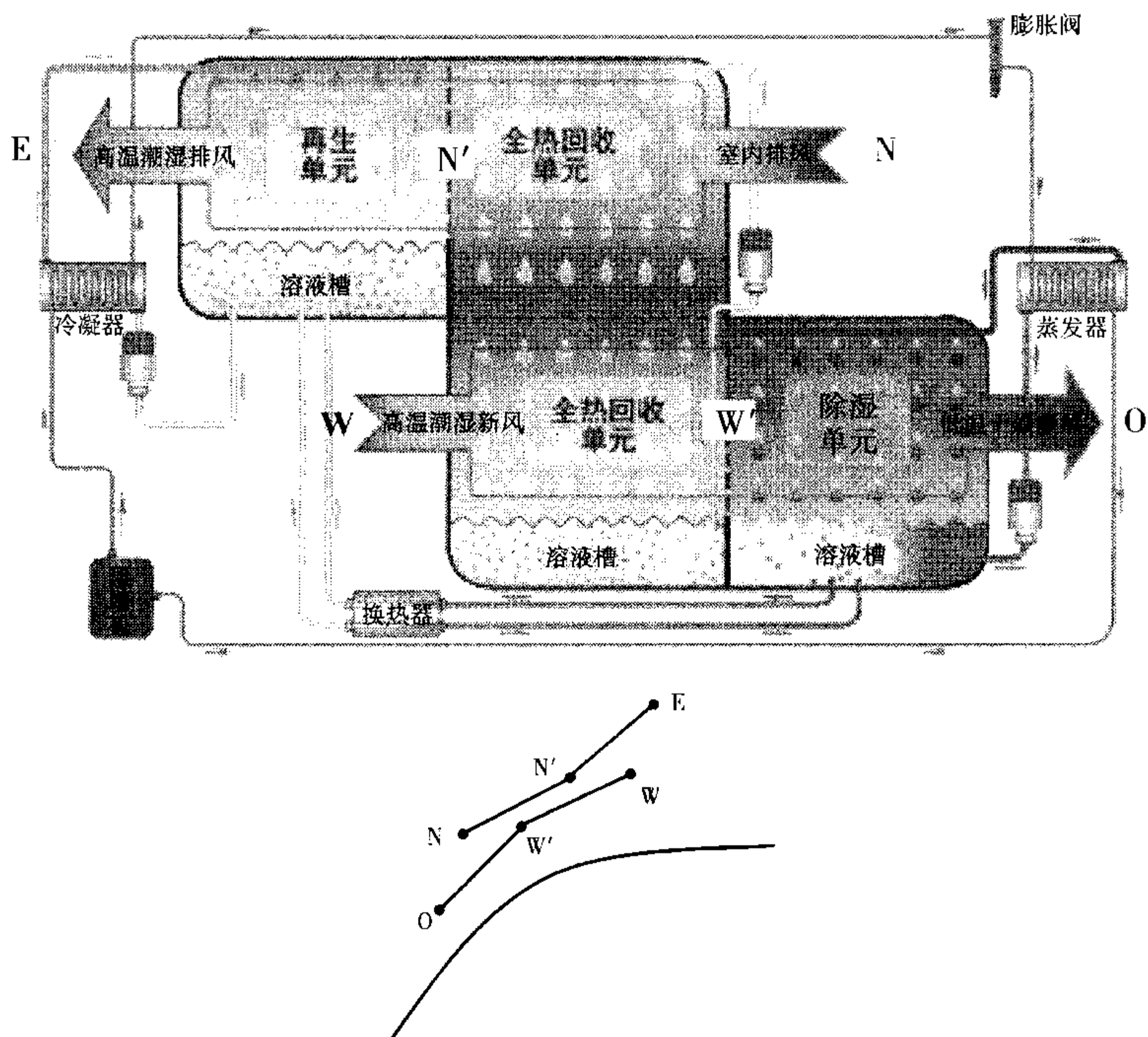
图 5. 17. 4 - 7 热泵驱动式溶液除湿系统
