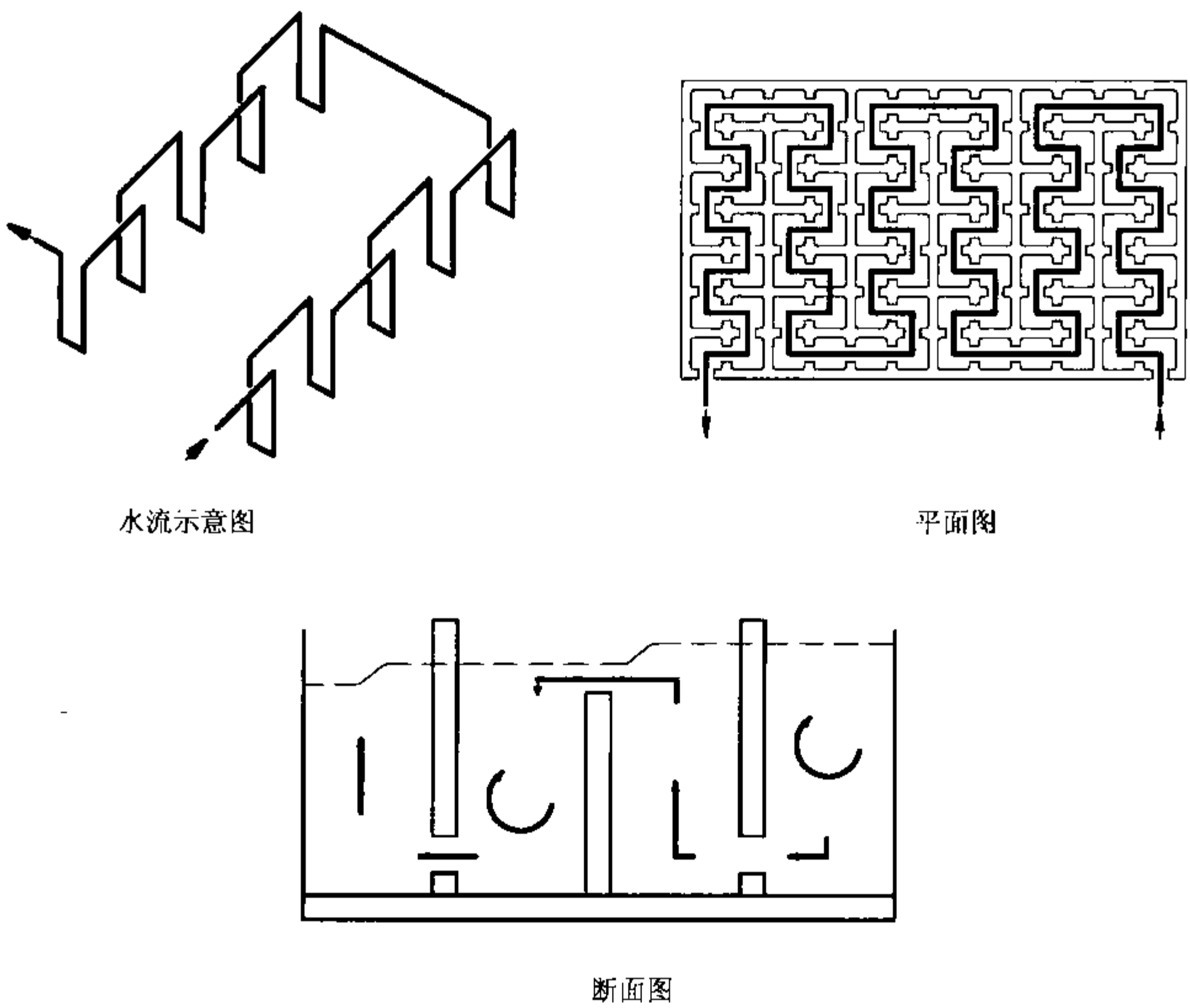
图 6.4.16-3 迷宫式蓄冷罐示意图
